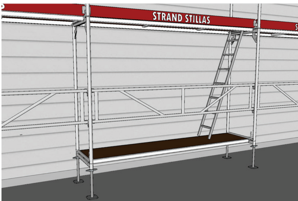
Fig. 17. Understøttelse av stige
