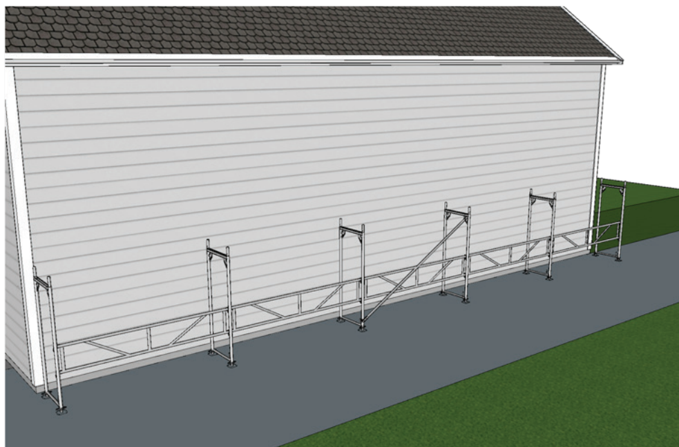
Fig. 12: Rammer og rekkverk montert på grunnplan
