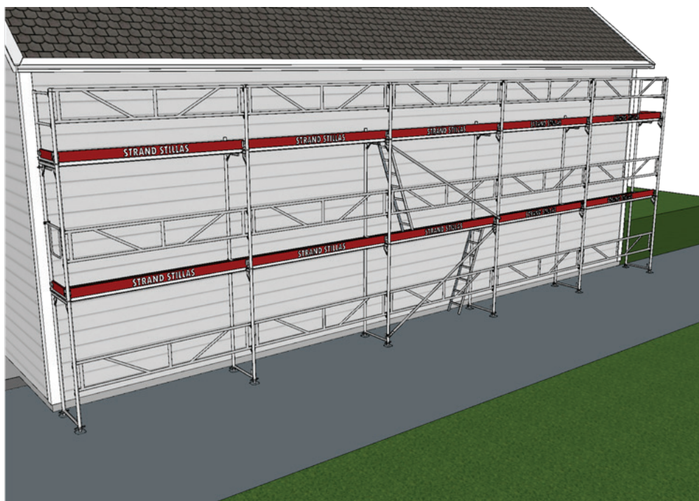
Fig 32: Monter låsesplinter og sparkebord.
