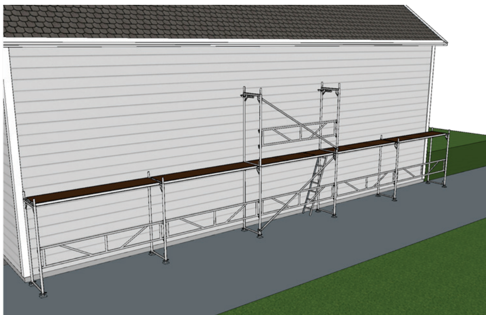
Fig. 18. Første stillasfag i 1. etg.
