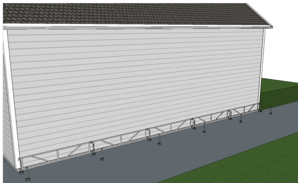
Fig. 7: Utlegging av spindelføtter
