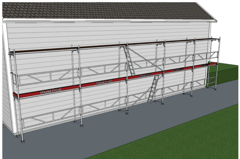
Fig. 28. Stillasgolv monteres deretter. Stigeoppgang monteres fortrinnsvis i samme stillas fag som i etasjen under, men med motsatt gangretning.
