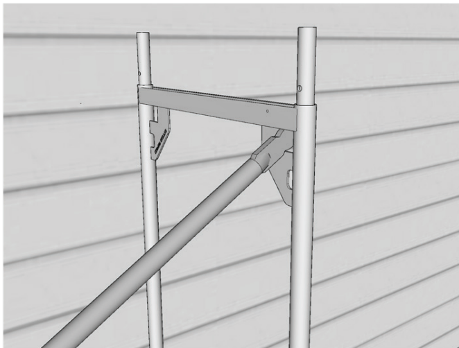
Fig. 9 og 10: Innfesting av diagonalstag i rammens øvre hjørne
