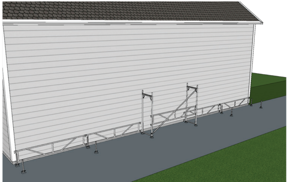
Fig. 8: Montering av første stillasfaget
