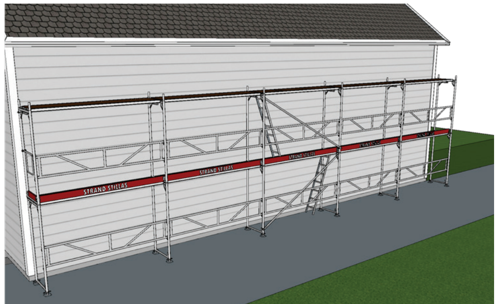
Fig. 24. Monter sparkebord.
