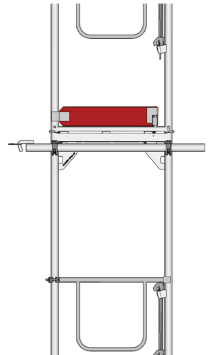
Fig. 37: Lang forankring
