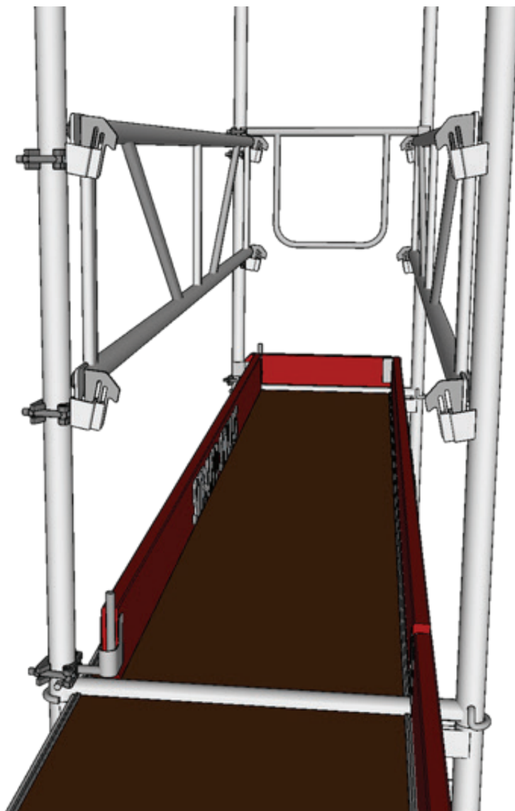
Fig. 41: Innvendig rekkverk
