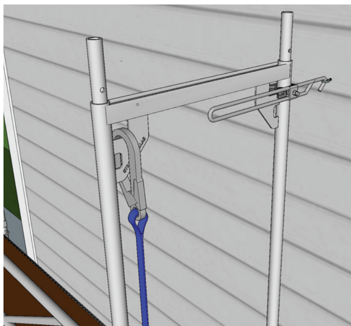
Fig. 47 Feste av fallsikring i øvre hjørne.
