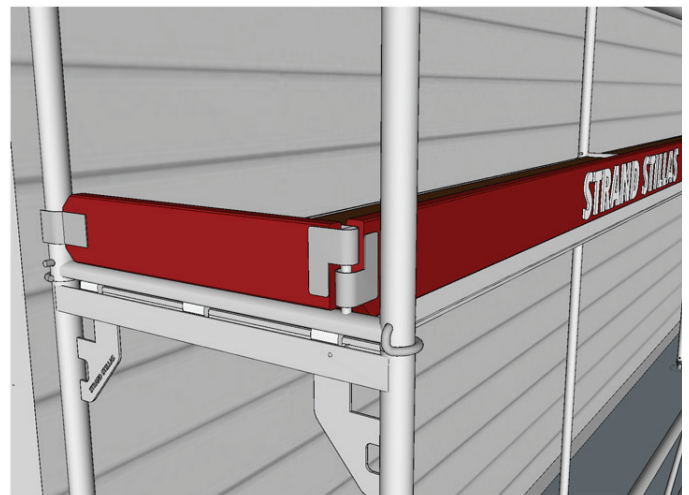
Fig. 25, 26, 27. Sparkebordene monteres i leseretningen sett fra stillasets innside ( montørens side). Det skal også monteres sparkebord i enden av stillaset.
