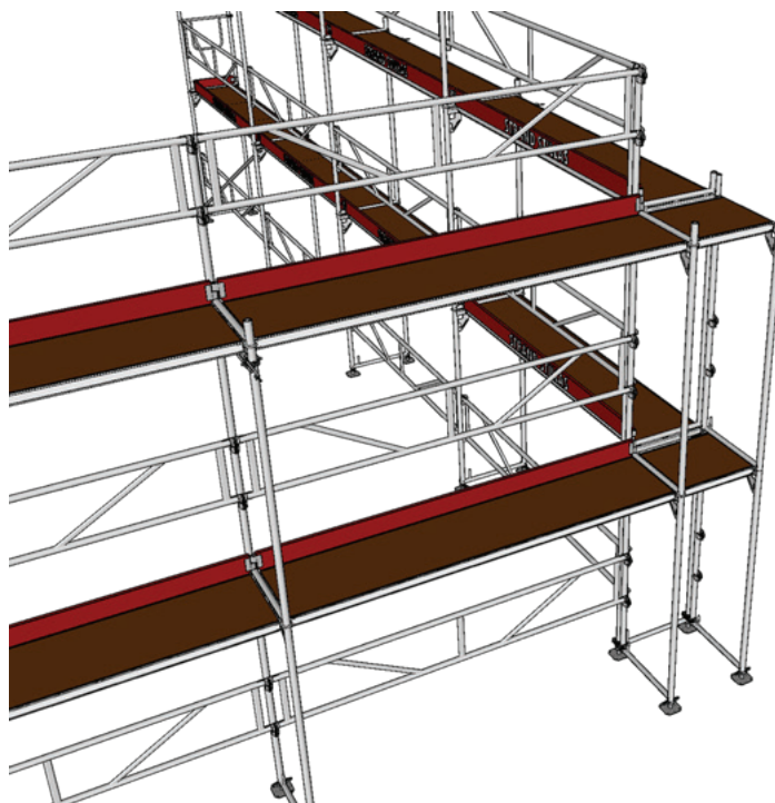
Figur 34: Innvendig hjørneløsning
