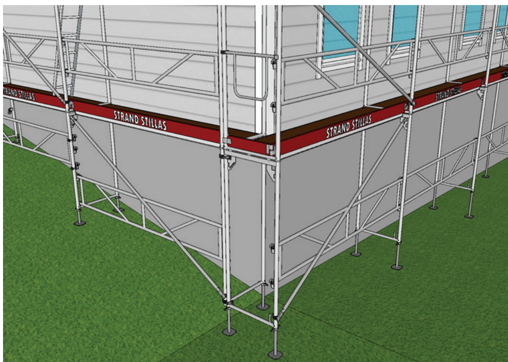
Fig. 33: Utvendig hjørneløsning
