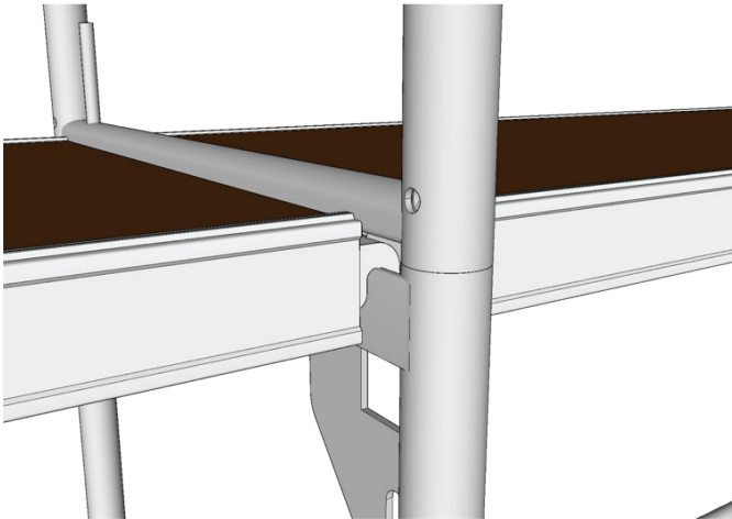
Fig. 22 og 23. For å sikre at rammene er skikkelig forbundet, samt å hindre uønsket utløfting av stillasgulva, monteres låsesplinter i rammenes nedre hjørne.
