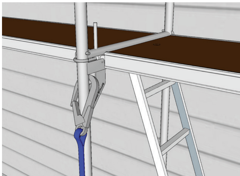
Fig. 46. Feste av fallsikring i øvre hjørne ved overgang til nytt nivå.
