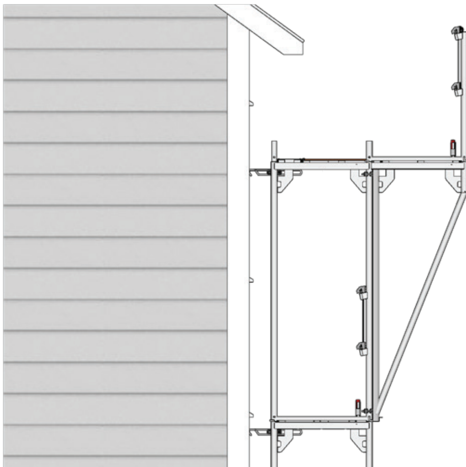
Fig. 40: Utvendig konsoll 0,73 m
